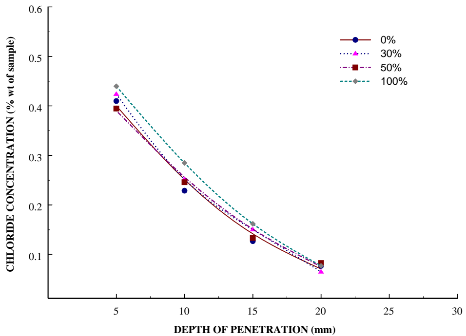
(b) PAV2 chloride diffusion profile.
