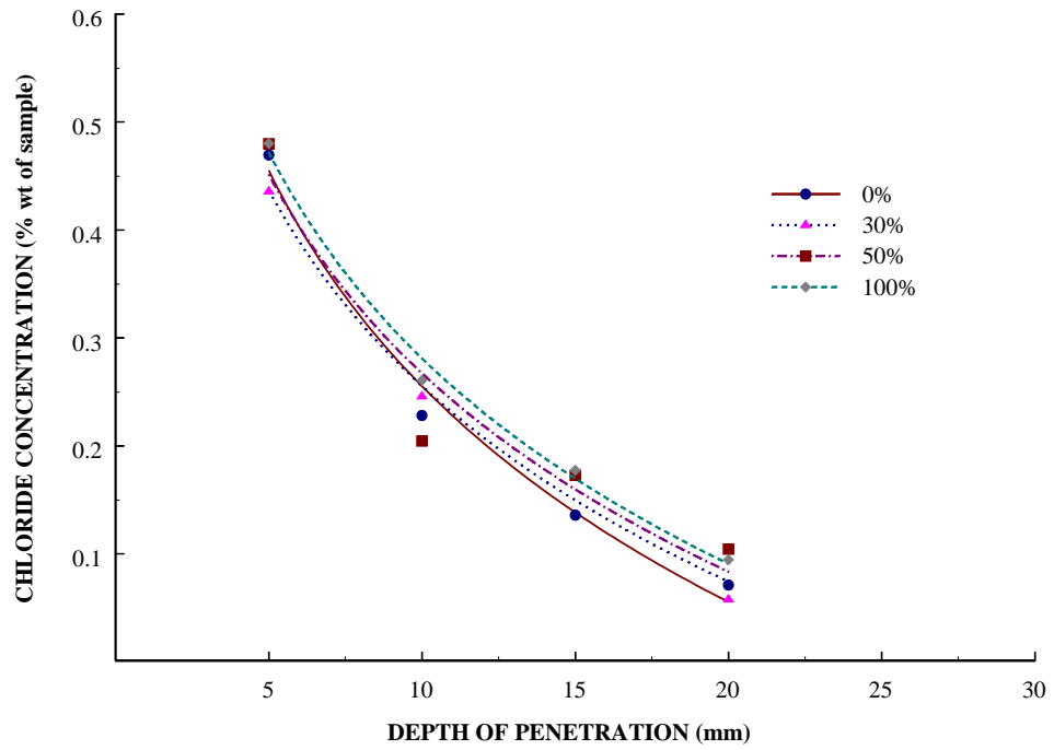
(a) PAV1 chloride diffusion profile.
